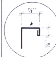
S-12 'J' trim
